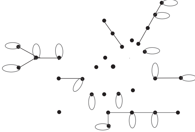
FIG. 5.8. The forest T - Q
